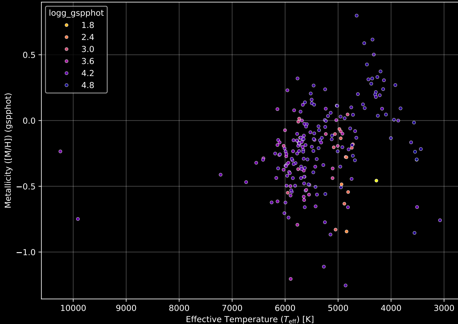
APOGEE DR17 Field: [170-60] Stellar Population Parameters (n= 219)
